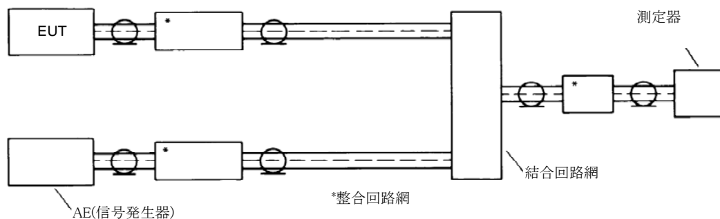
図 C.8—TV/FM 放送受信機チューナポートにおけるエミッション電圧の測定のための接続配置
