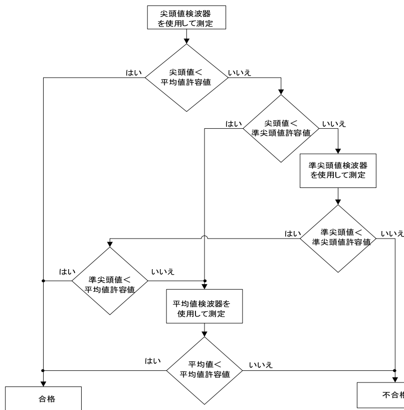
図 C.3—準尖頭値及び平均値許容値に関する各種検波器を用いるための判定ツリー
