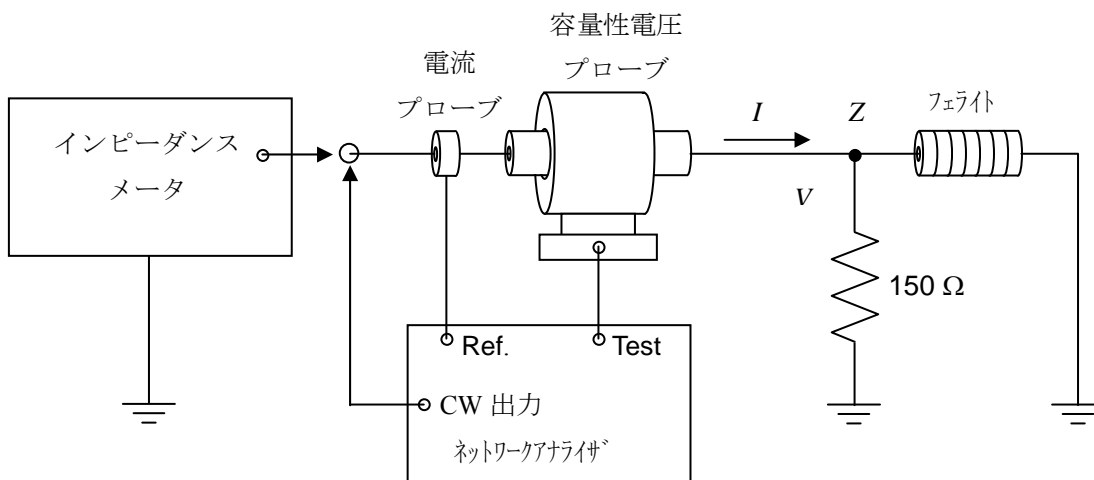
図 G.15— 150 \Omega とフェライトによる合成インピーダンスの基本測定配置
