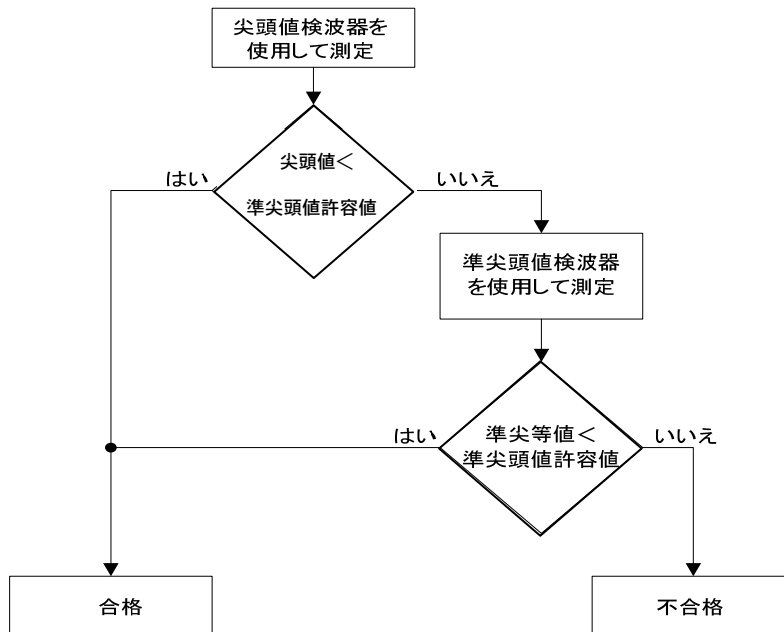
図 C.5—準尖頭値許容値に関する各種検波器を用いるための判定ツリー
