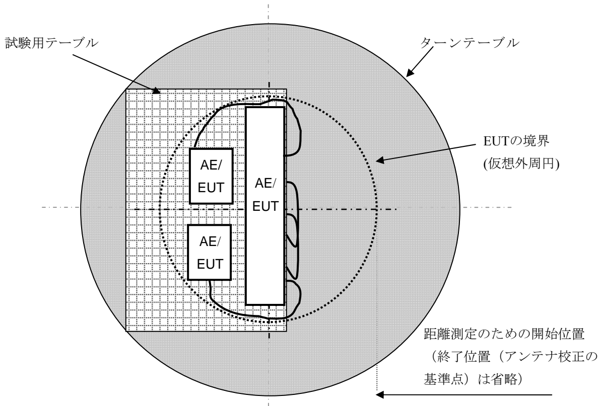
図 C.2—EUT, ローカル AE 及び関連ケーブルの境界
