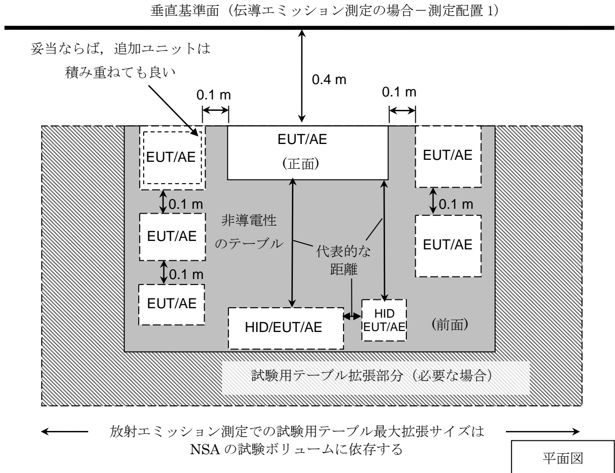
図 D.1－卓上型 EUT の測定配置例 （伝導及び放射エミッション）（平面図）
