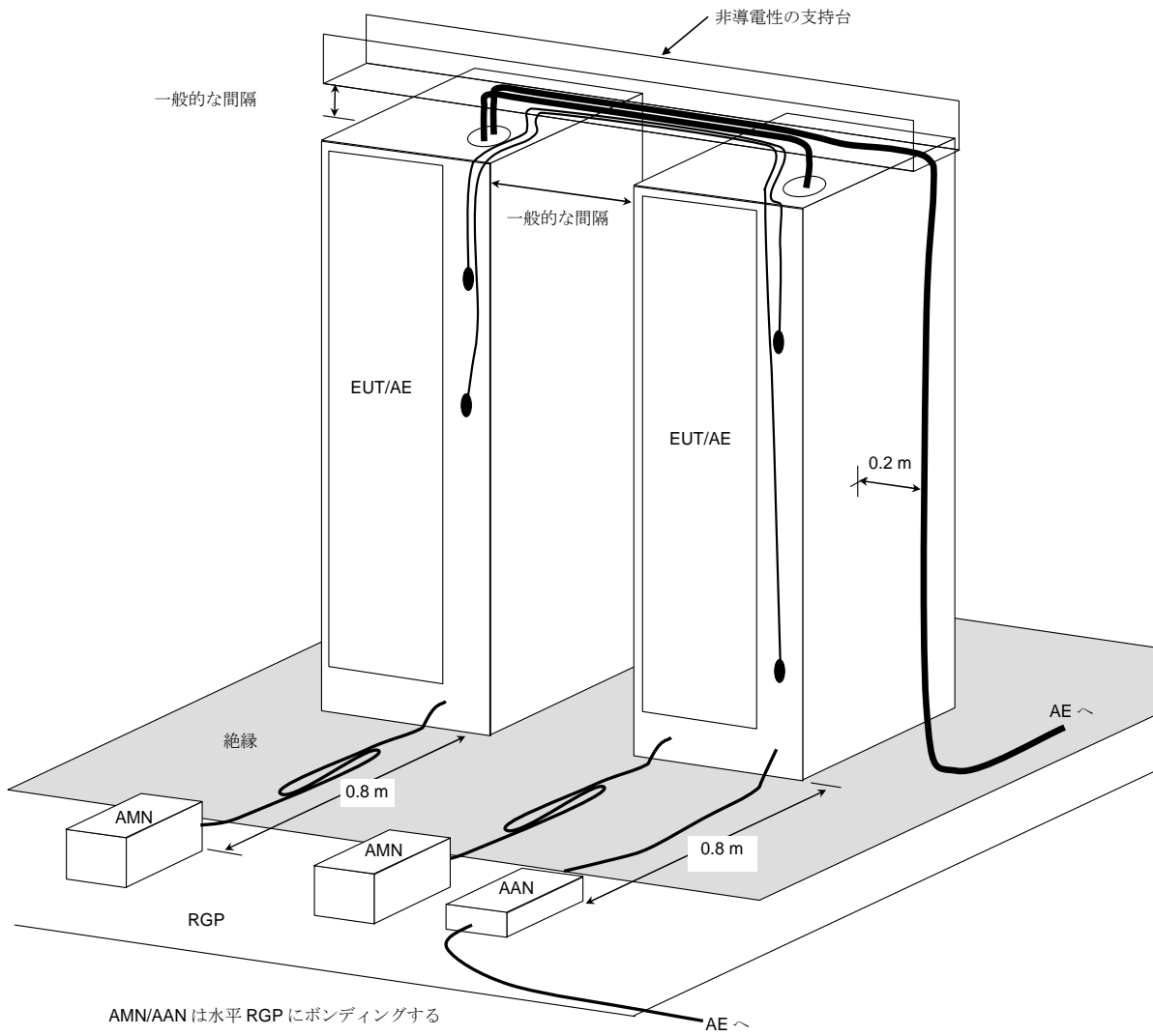
図 D.6—床置型装置の測定配置例（伝導エミッション測定）
