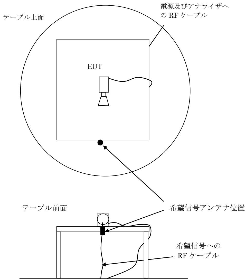
図 H.2—希望信号用送信アンテナの測定配置例
