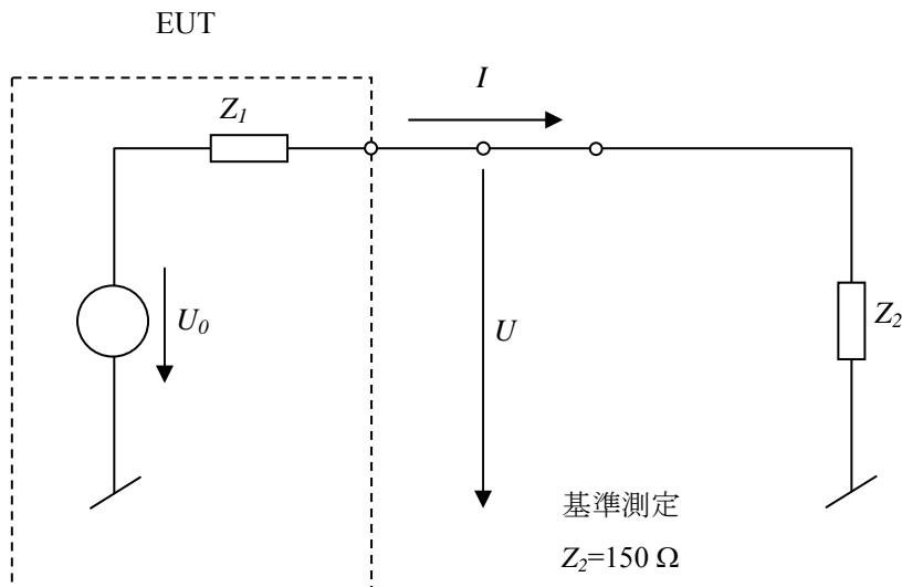
図 G.12—コモンモードインピーダンス 150 Ω で定義された許容値を考えるための基本回路
